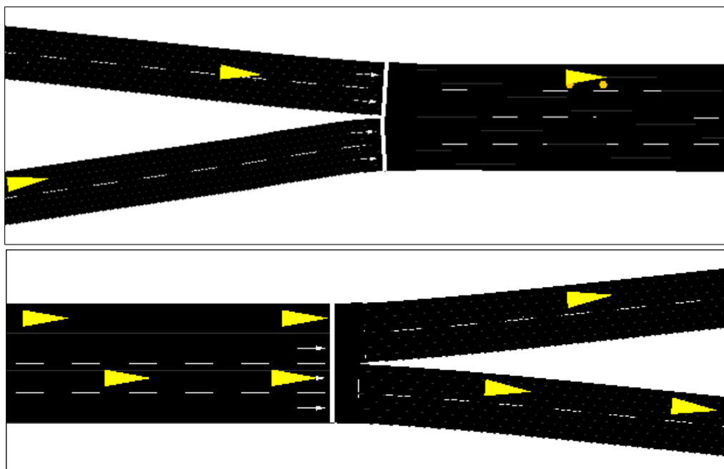
Obrázek 3. Scénář nájezdy a sjezdy – základní zobrazení nájezdu v simulačním nástroji SUMO
